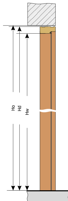
Wymiary ościeżnicy blokowej, system przylgowy
